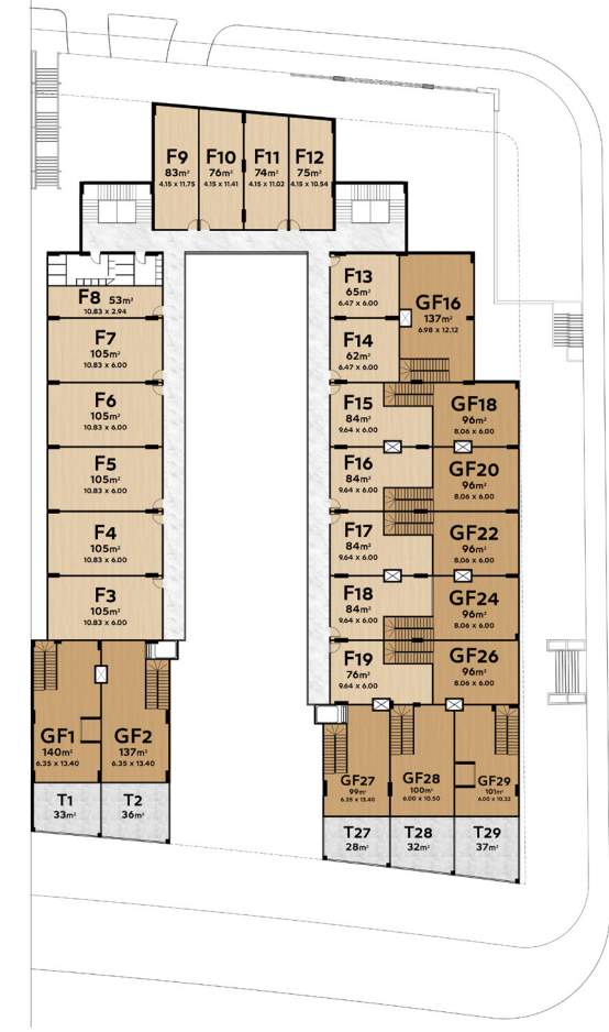
الدور الأول
